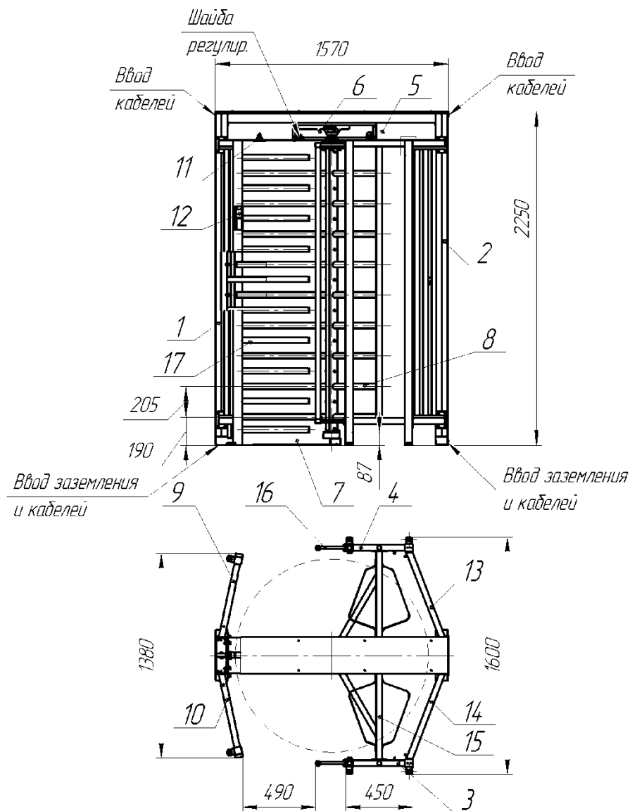
Габаритные размеры турникета «Ростов-Дон ПР1Ш/3М2»
